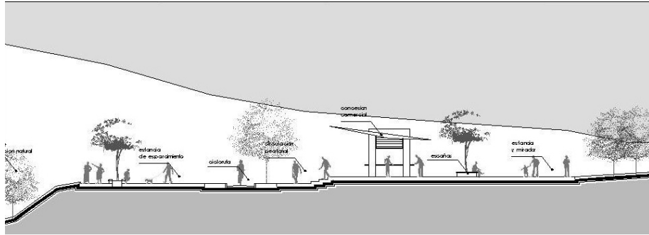
CORTE ALAMEDA ESTRUCTURANTE ESC. 1:200
